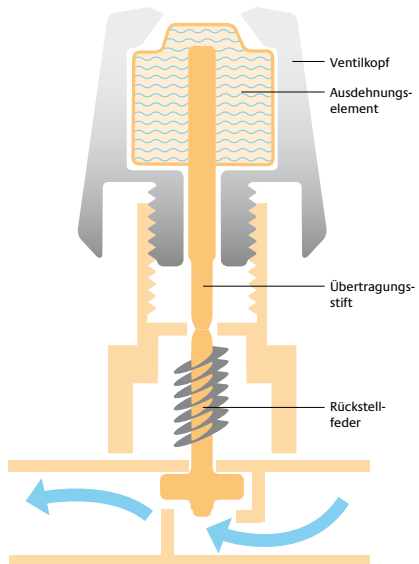
Aufbau eines Thermostatventils
